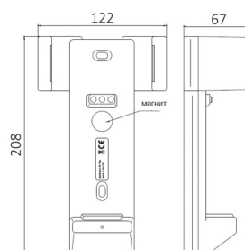
Пост зарядки ASN15HD
