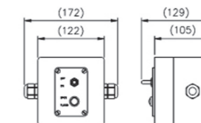
Пульт дистанционной регулировки луча накладного монтажа для LX300 D и C
