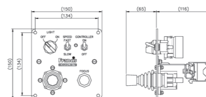
Пульт дистанционного управления (джойстик) для LX300RC
