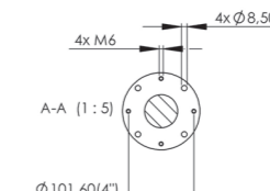
Данные для монтажа основания RC
