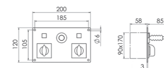
RCU-E пульт дистанционного управления (встраиваемый)
