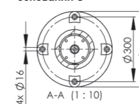
Данные для монтажа основания CP
