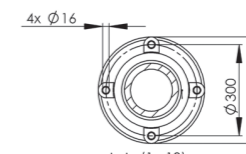
Данные для монтажа основания DP
